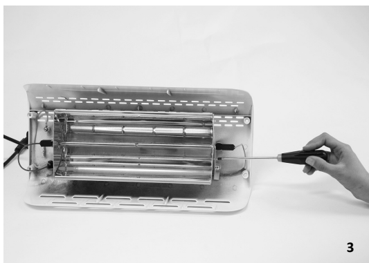
3. SVITARE LE VITI CHE TENGONO LE DUE PICCOLE PROTEZIONI LATERALI.
