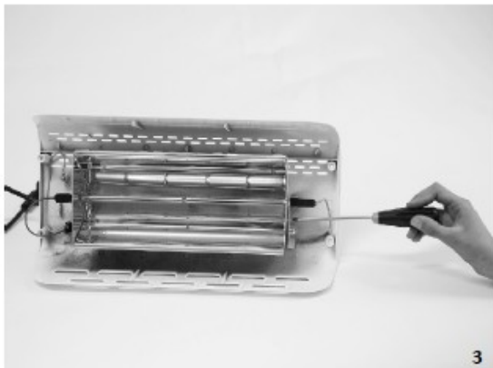
3. DÉVISSER LES VIS QUI TIENNENT LES DEUX PETITES PROTECTIONS LATÉRALES.
