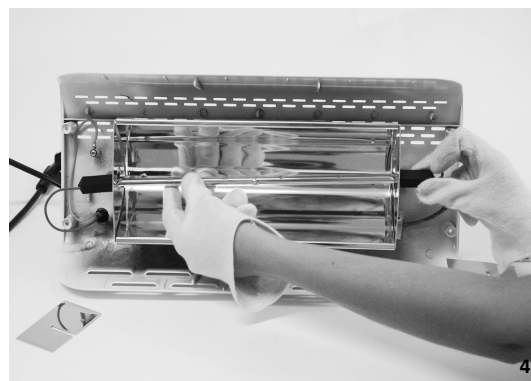
4. ESTRARRE IL BULBO DALLE MOLLETTE
