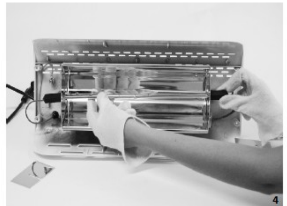
4. EXTRAIRE L'AMPOULE DES CLIPS
