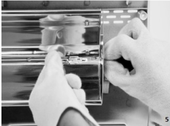
5. ÔTER LES DEUX PROTECTIONS THERMO-ÉLASTIQUES QUI RECOUVRENT L'EXTRÉMITÉ DE L'AMPOULE ET DÉCONNECTER LES DEUX COSSES (FASTON) QUI RELIENT LES FILS D'ALIMENTATION À L'AMPOULE (SI LES PROTECTIONS SONT ABÎMÉES, IL FAUT LES RETIRER EN COUPANT LES FILS D'ALIMENTATION PRÈS DES DEUX COSSES (FASTON))
