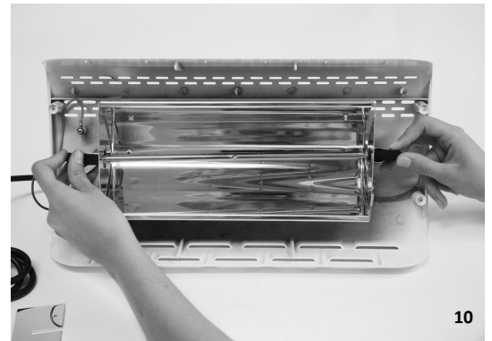
10. RICOMPORRE L'APPARECCHIO PROCEDENDO ALL'INVERSO.
