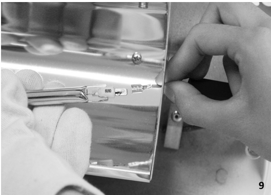
9. CONECTAR LOS FASTON MACHOS DE LA NUEVA BOMBILLA CON LOS DE LOS DOS CABLES, REVESTIRLOS CON LAS CÁPSULAS Y VOLVER A COLOCAR LA BOMBILLA EN LA SEDE DE LOS RESORTES.
