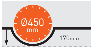
MAX. SCHNITTIEFE - P13
